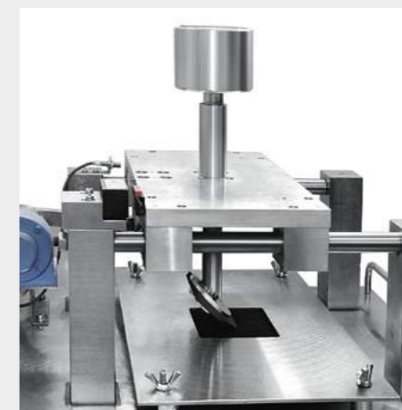
Heel test device
